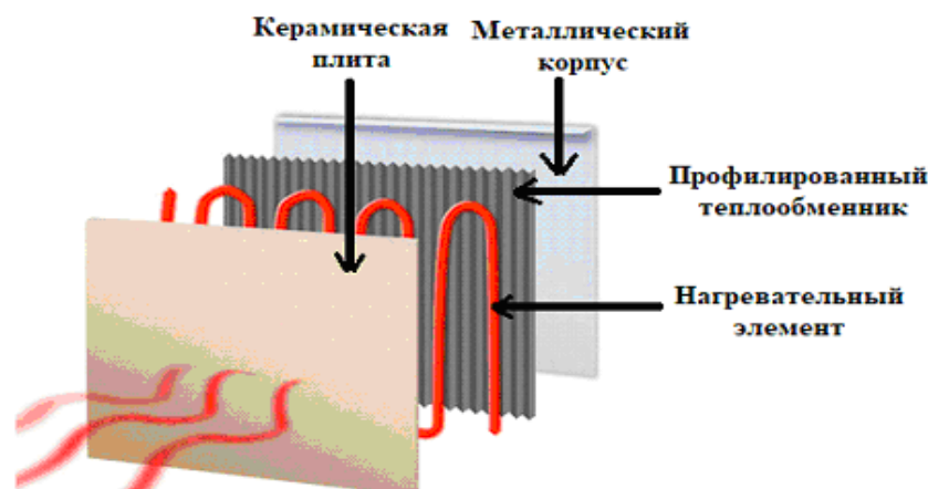
Рис. 1. Керамическая инфракрасная панель
