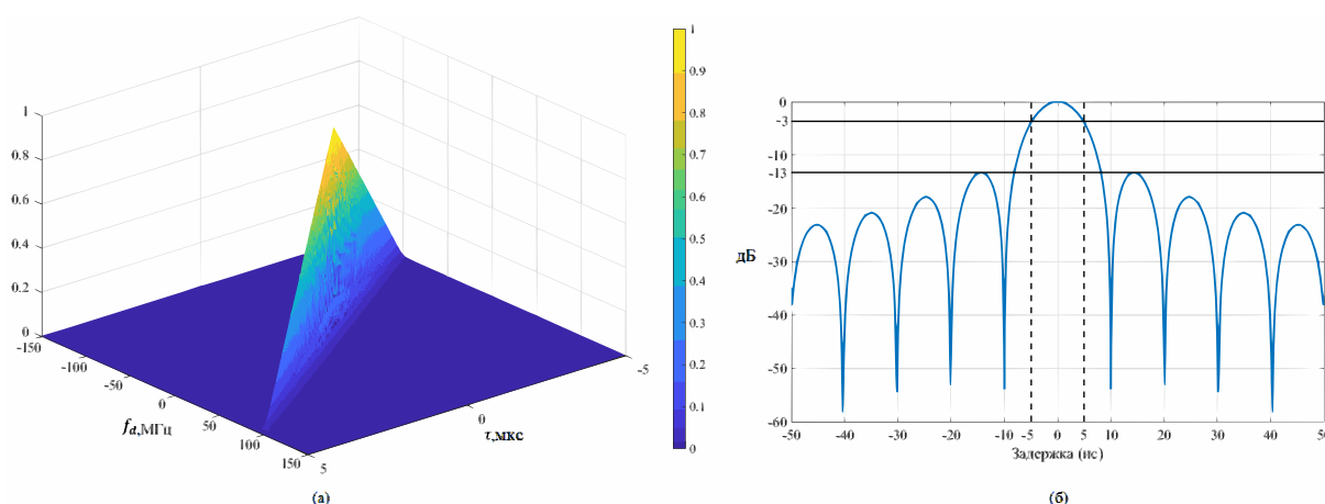
Рис. 3. Вид тела ФН ЛЧМ сигнала длительностью 5 мкс (а), вид сечения тела ФН при f_d = 0 (б)
