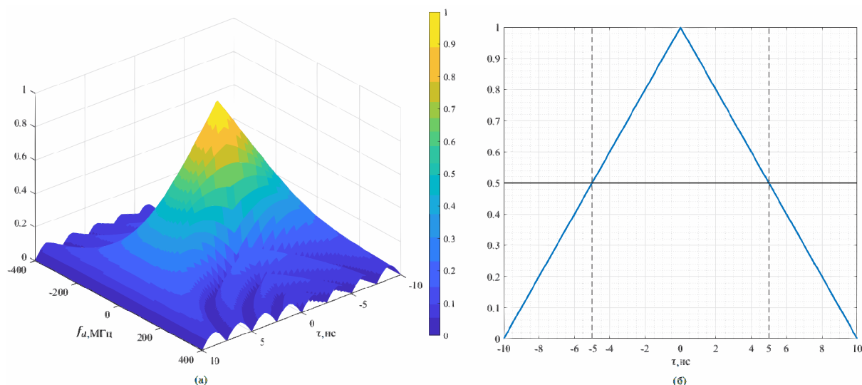
Рис. 1. Вид тела ФН прямоугольного импульса длительностью 10 нс (а), вид сечения тела ФН при f_d = 0 (б)
