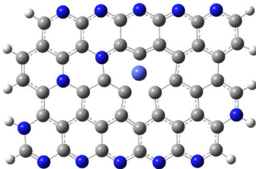
Рис. 1. Расположение атомов металла над поверхностью ППАН
