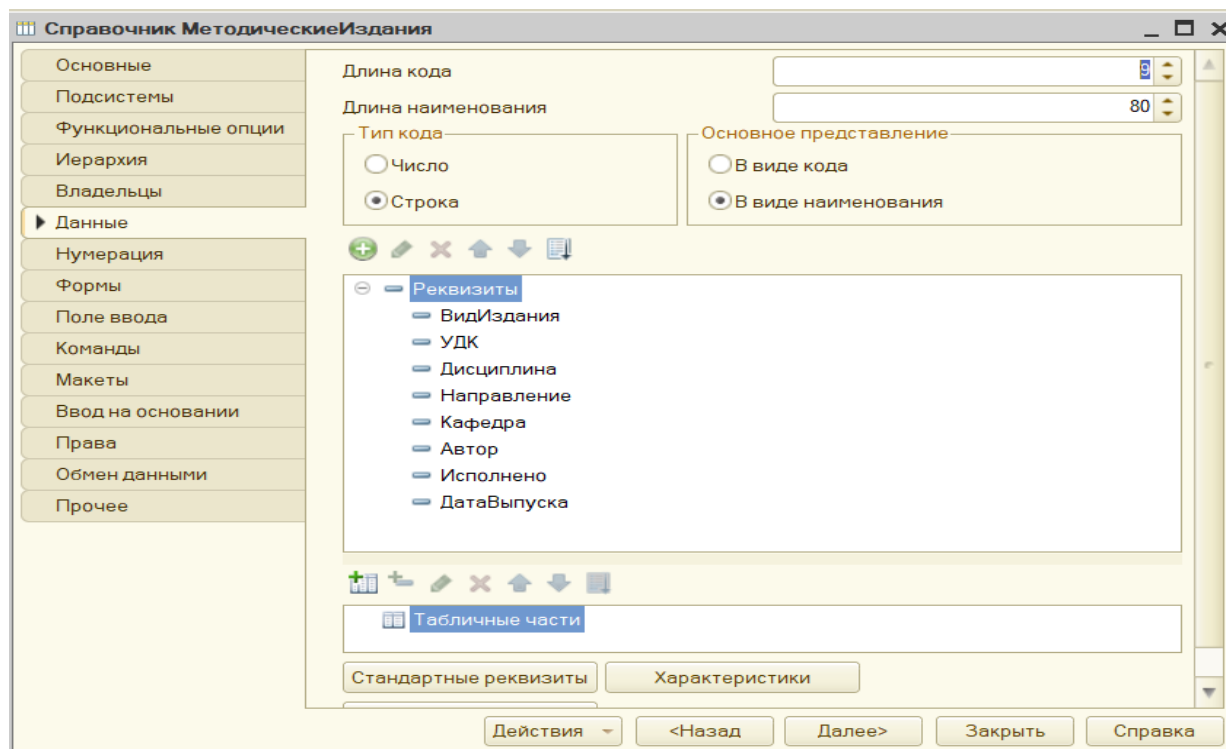
Рис. 2. Структура справочника «Методические издания»
