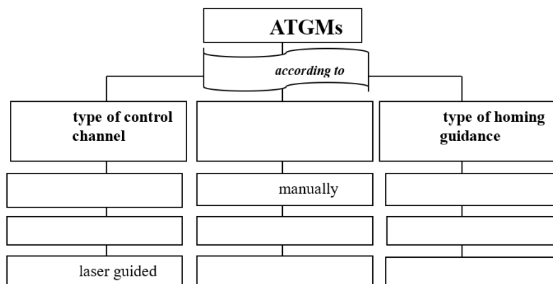
Рис. 1. Классификация ПТУР
