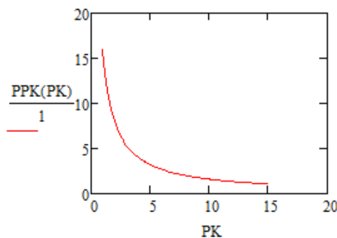
Рис. 1. График давления конденсации дистиллята по графику функции изотермы паровой фазы
