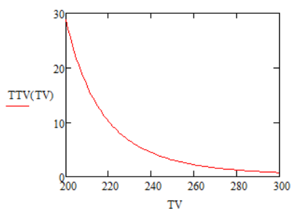
Рис. 2 – График температуры верха колонны
