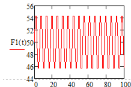
Рис. 6. График импульсного изменения питания
