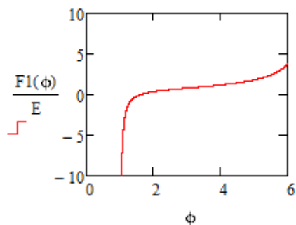
Рис. 5. График флегмового числа по методу Андервуда
